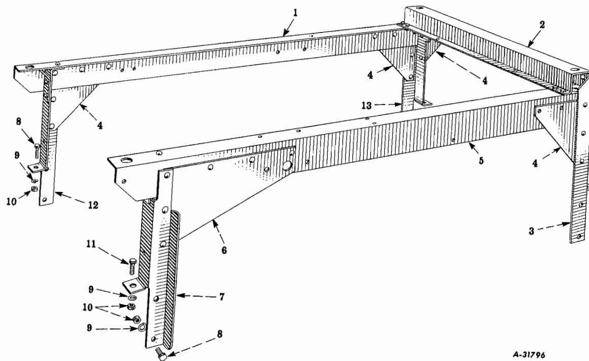
FIG. 16-7 - CAB SUB FRAME (For Cab Codes 1606, 1613) (RC-160)
